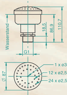
dysza Wulkan 37-2,5 kod 4821050
